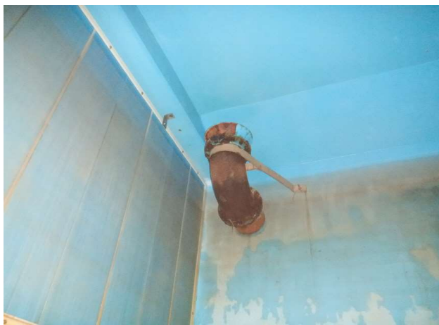
배수지 1지 유입배관 관부식
