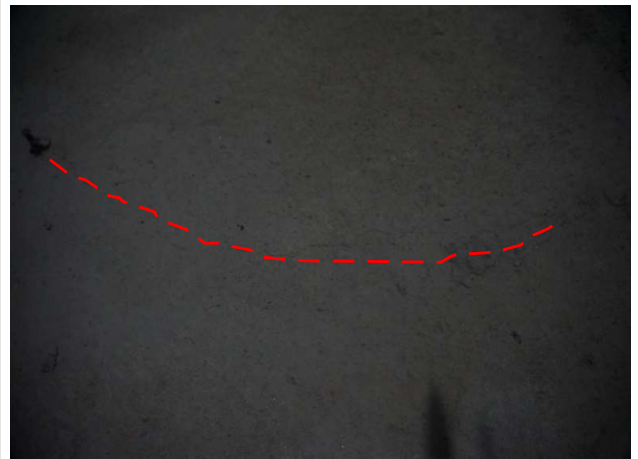
유출밸브실 하부슬래브 균열(0.3mm미만)
