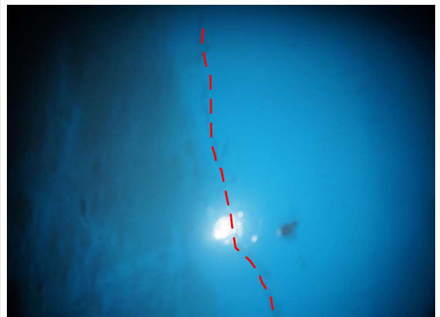
배수지1지 하부슬래브 균열(0.3mm미만)
