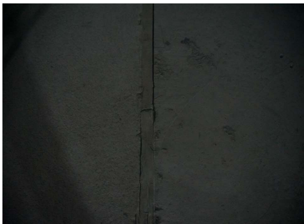
유입밸브실 상부슬래브 시공이음부 실링재 파손
